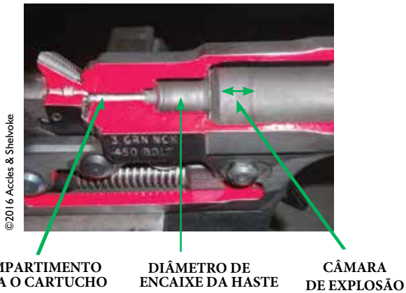
Fig. 8.04 Haste de limpeza em uso numa CASH Special
